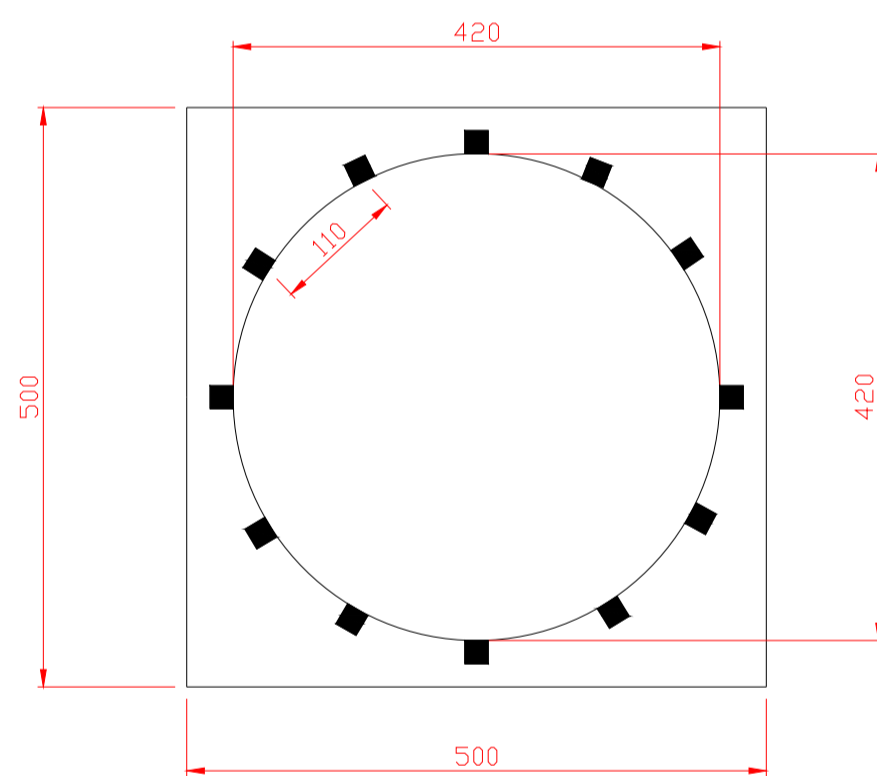
PLANTA BAIXA
