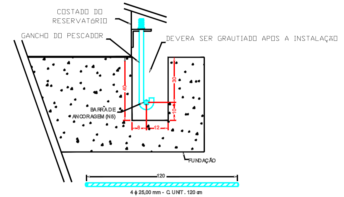
DETALHE DOS CHUMBADORES
