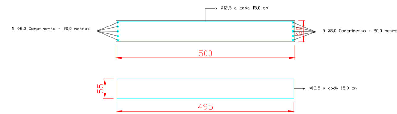
ARMAÇÃO DA BASE
